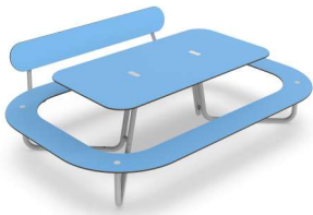
Plateau O, L ja I: pituus: 273 cm syvyys: 183 cm korkeus: 73 cm
